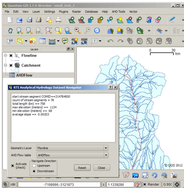
Figura A-5. El Navegador RTI Analytical Hydrology Dataset mostrando la navegación aguas abajo de la línea de flujo
