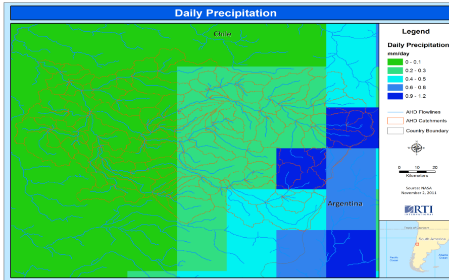
Figura 8. Precipitación indexada a cuencas de la AHD
