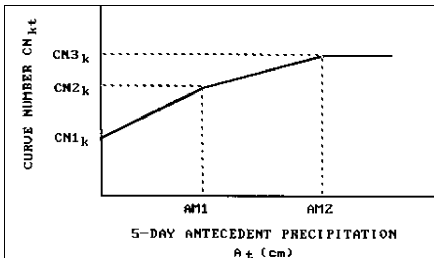
Figura 3. Los números de curva se seleccionan como funciones de la humedad antecedente, como se describe en Haith (1985).
