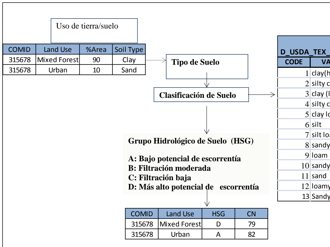
Figura 5. Representación esquemática de la estimación del número de curva. El ejemplo aquí dado es para una sola Cuenca de la AHD COMID=315678 que tiene dos tipos de usos de tierras (Bosque mixto y Urbano) y cada uso de tierra tiene un solo tipo de suelo dominante.
