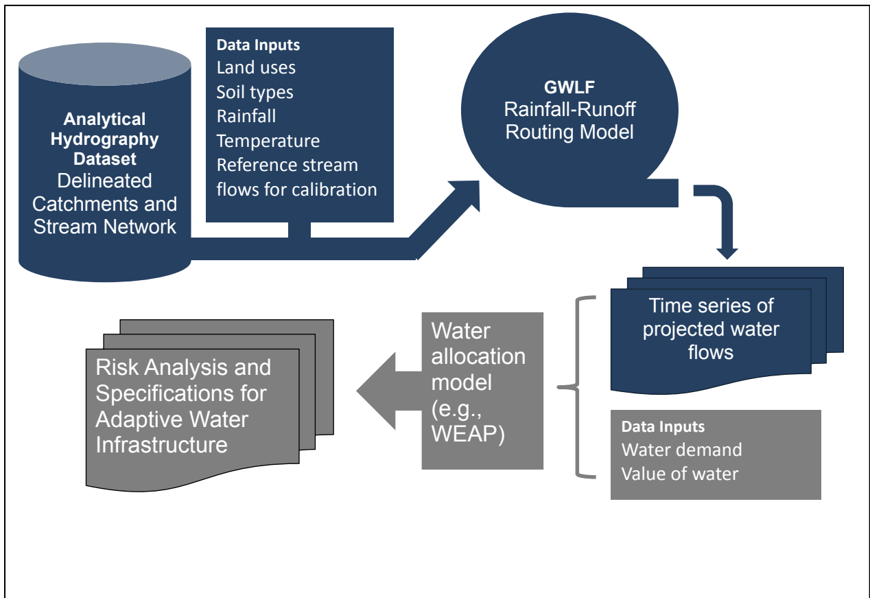
Figura 1. Diagrama de Flujo del Hydro-BID
