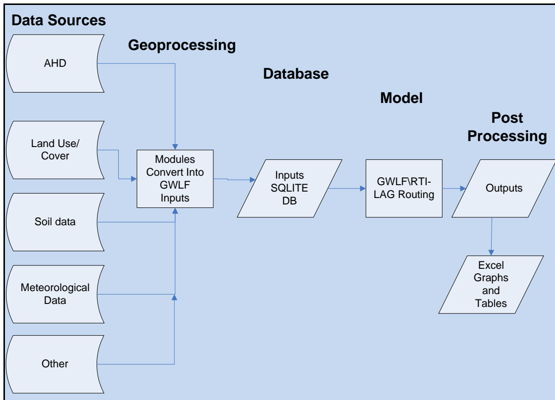
Figura 10. Flujo de datos
