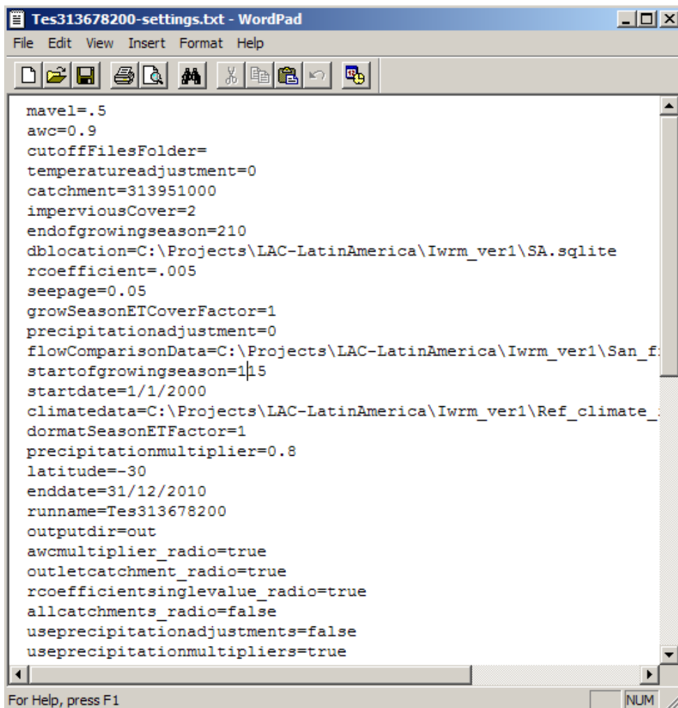
Figura 19. Archivo setting
