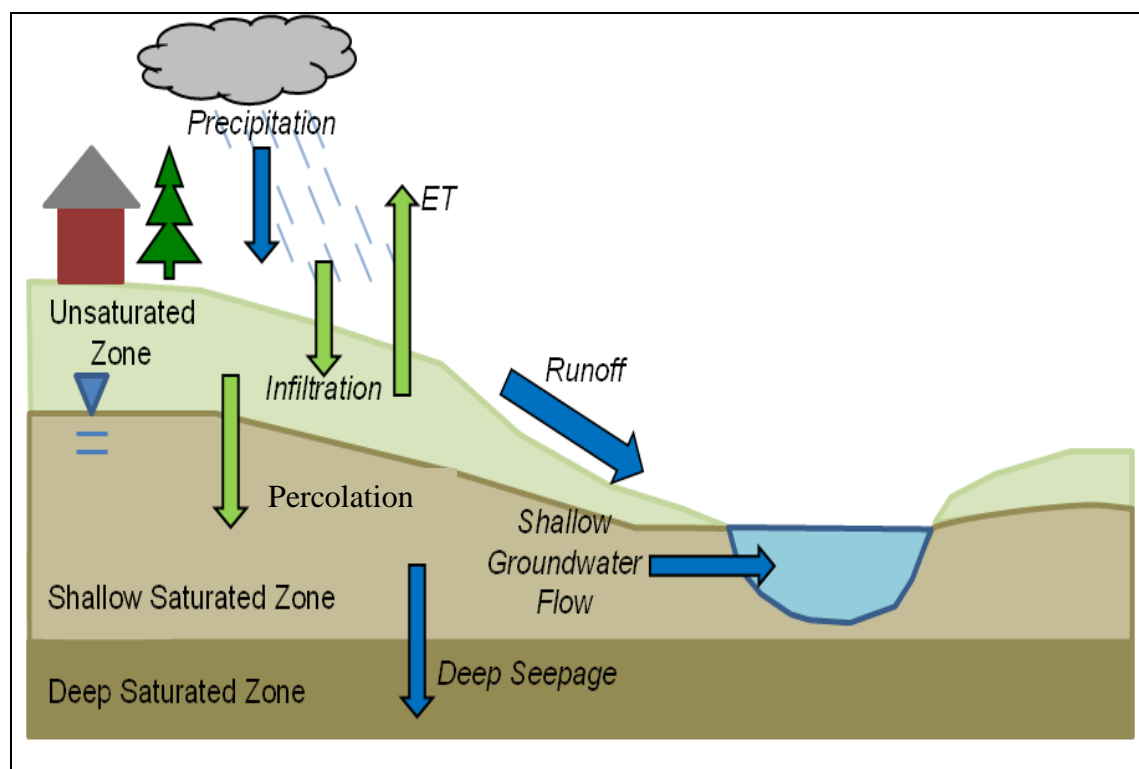
Figura 2. La representación esquemática del modelo de GWLF (modificado de Haith et al., 1996).
