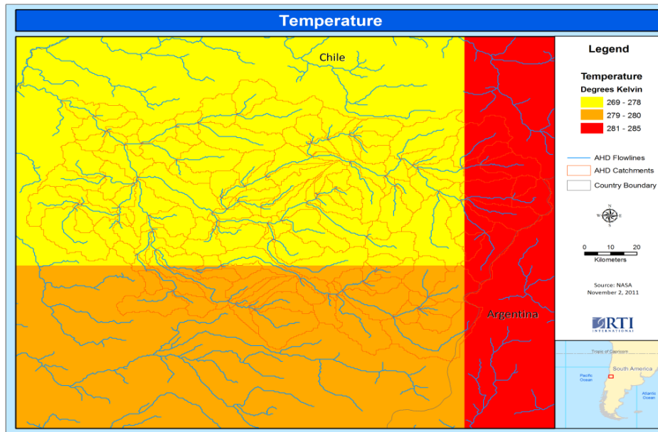
Figura 9. Temperatura indexada a cuencas de la AHD
